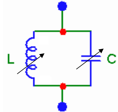
Rinnakkaisresonanssiipiiri (Resonanssissa oleva taajuus ei mene "läpi")
